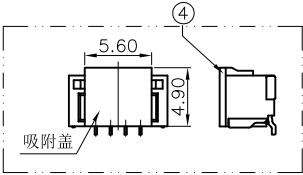
产品装上吸盖示意图 SCALE 1:2
