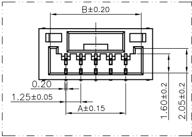
6PIN及以下示意图
